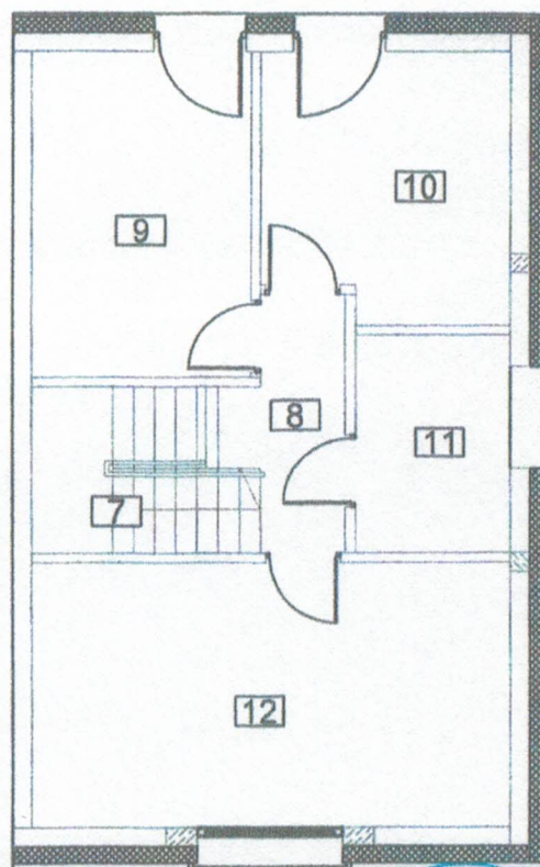
Rzut piętra
