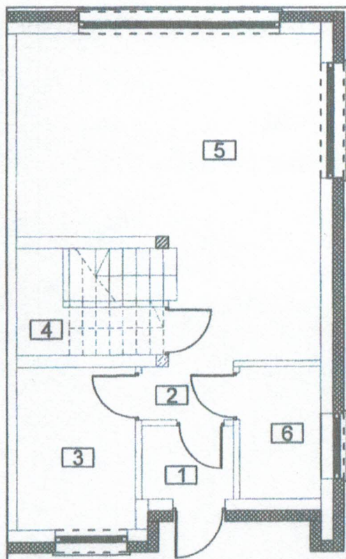
Rzut parteru
